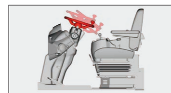
チルト&テレスコピック機能付きステアリングホイール ポップアップステアリングコラムとペダル
